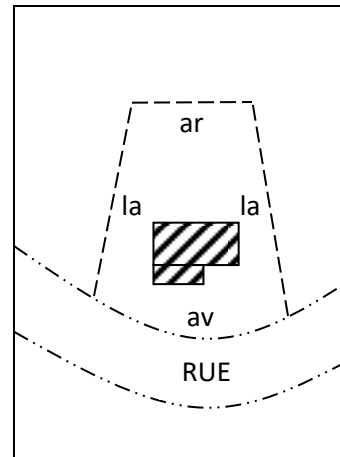
LOT À L'INTÉRIEUR D'UNE COURBE
